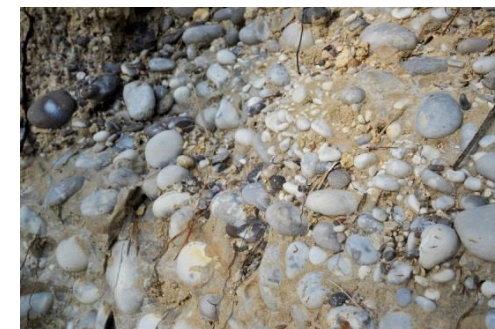
Poudingue
