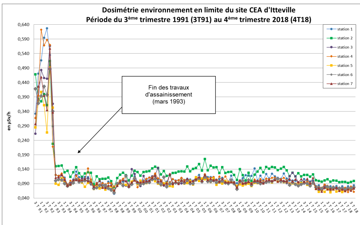
Figure n°4 - Évolution du débit de dose horaire moyen (3 ème trimestre 1991- 4 ème trimestre 2018) en limite du site d'Itteville.
